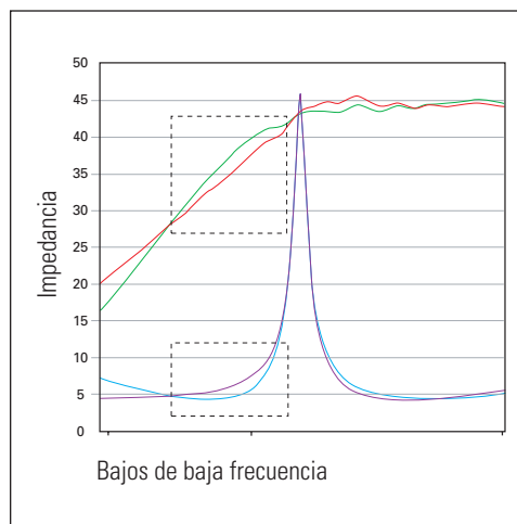
ACOPLAMIENTO CAPACITIVO
