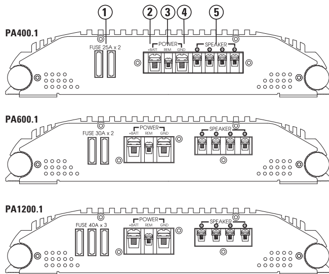
ABILDUNG 3—VERSTÄRKERANSCHLÜSSE—HINTEN (PA400.1/PA600.1/PA1200.1)
